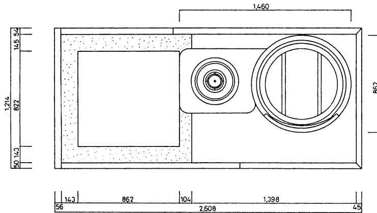
図11 同かまど・囲炉裏平面図
