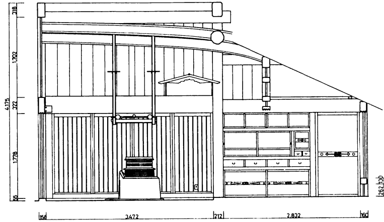
図9 同台所現状展開図(納戸境)
