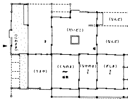
図6 北谷家住宅復原平面図(19c前期)
