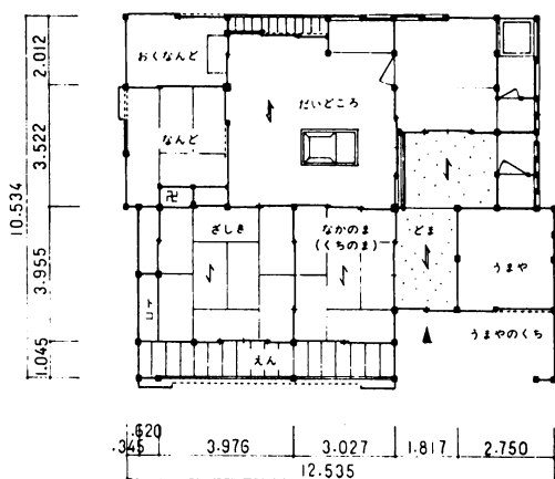
図3 清水家住宅現状平面図
