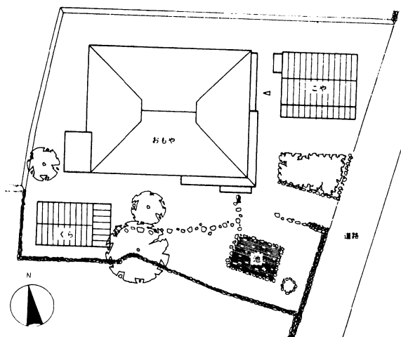
図2 大江家住宅配置図
