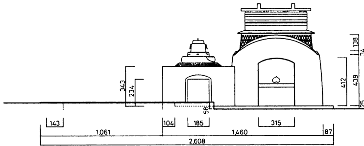
図10 同かまど・囲炉裏正面図
