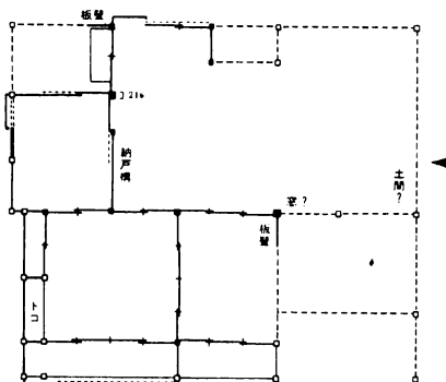
図5 同復原平面図(18c後期)
