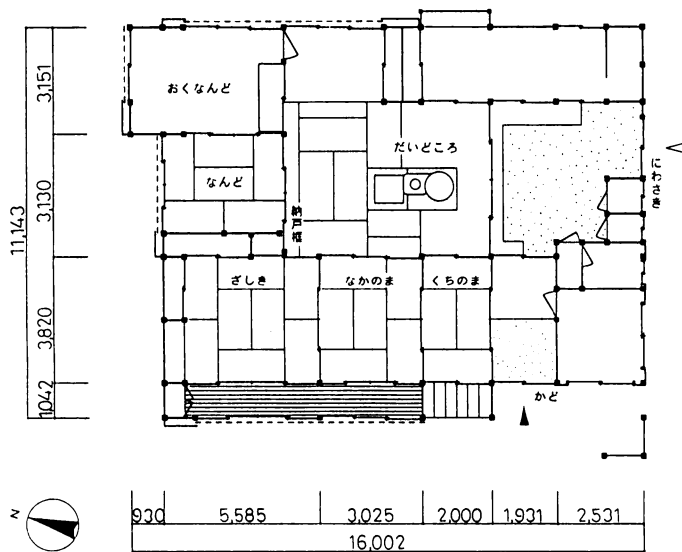
図8 檀林家住宅現状平面図
