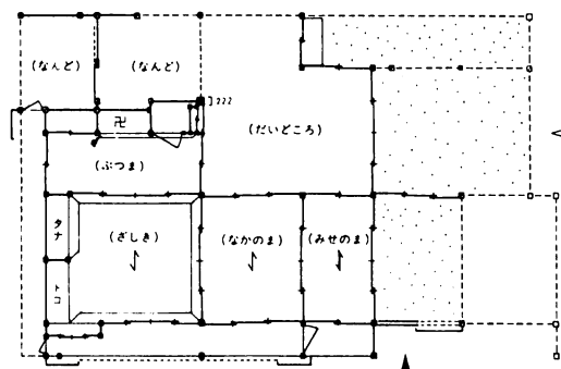
図7 山田家住宅復原平面図(19c 後期)
